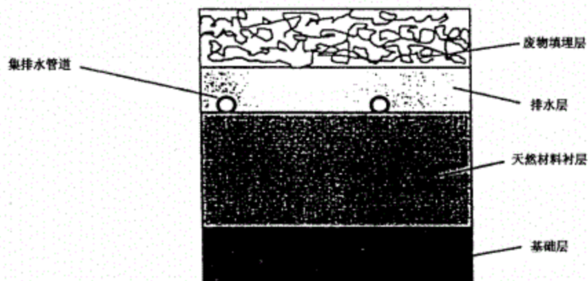
图 A.3 天然材料衬层示意图
