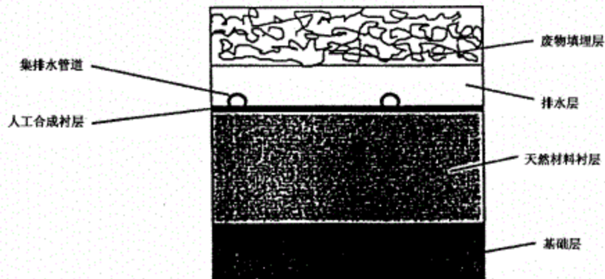
图 A.2 复合衬层示意图
