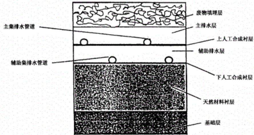
图 A.1 双人工衬层示意图
